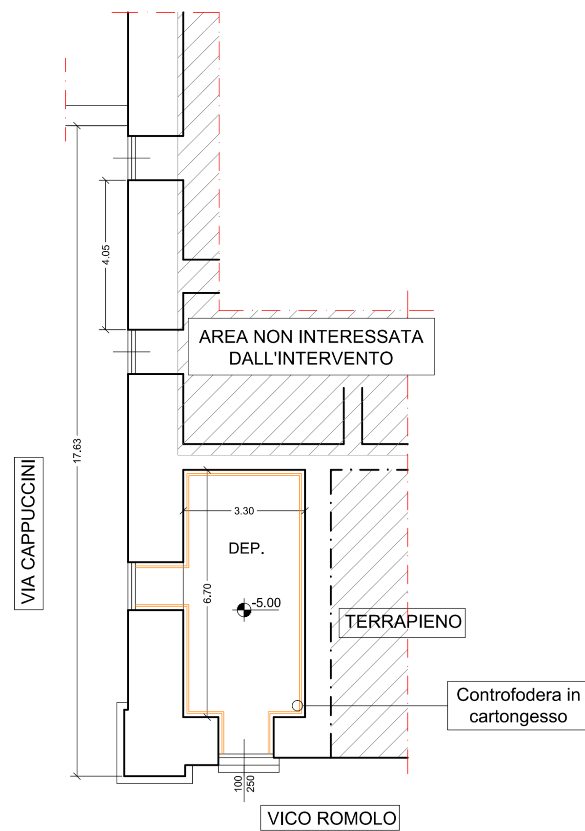
PROGETTO - PIANTE PIANO SEMINTERRATO PIANTE QUOTATA SCALA 1:100
